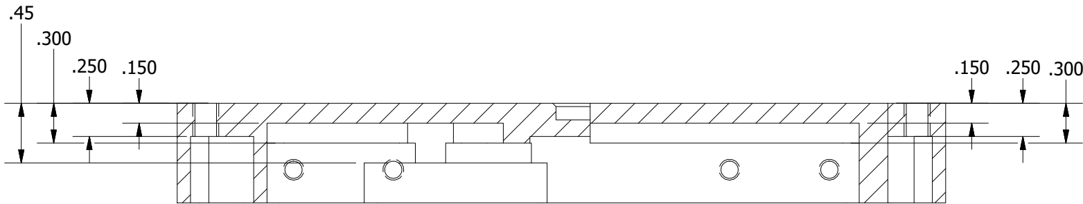
SECTION A-A
